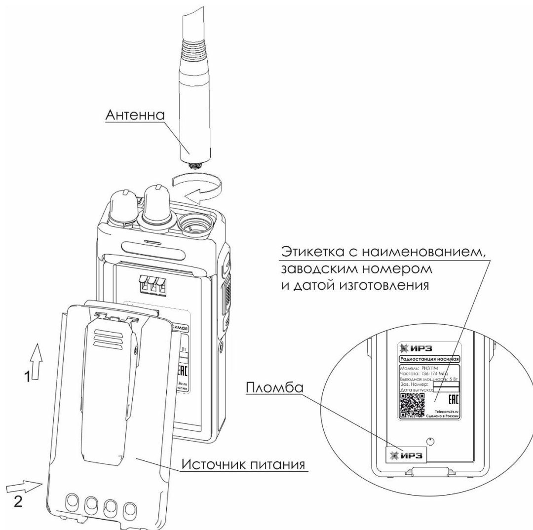
Рисунок 2.1 – Подключение антенны и источника питания к радиостанции
