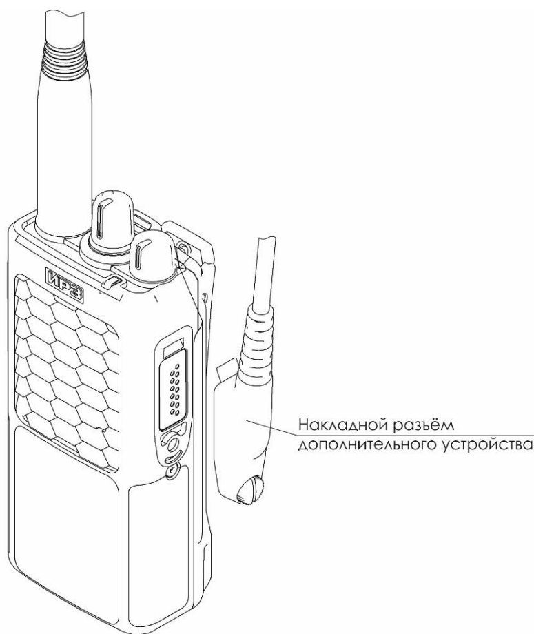
Рисунок 2.2 – Подключение дополнительного устройства к радиостанции
